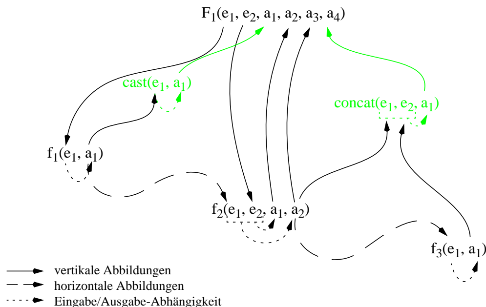
Abbildung 4: Funktionsabbildung mit zusätzlichen Funktionen zur Weiterverarbeitung der Parameter.
