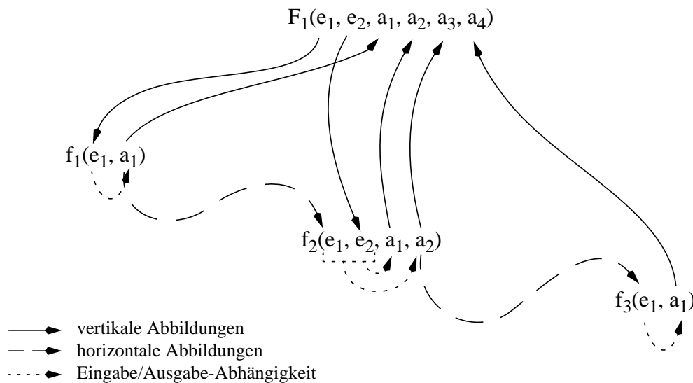
Abbildung 3: Abhängigkeiten der Parameter.
